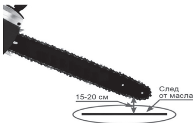
Рис. 9 Проверка подачи масла
